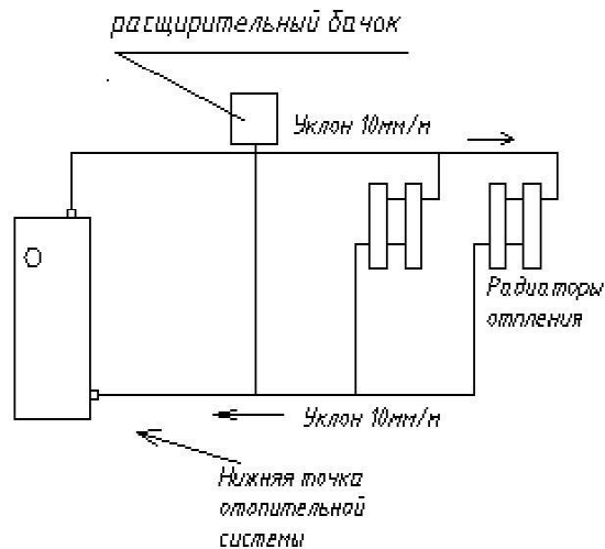
Рис.1 Схема монтажа открытой системы отопления.
